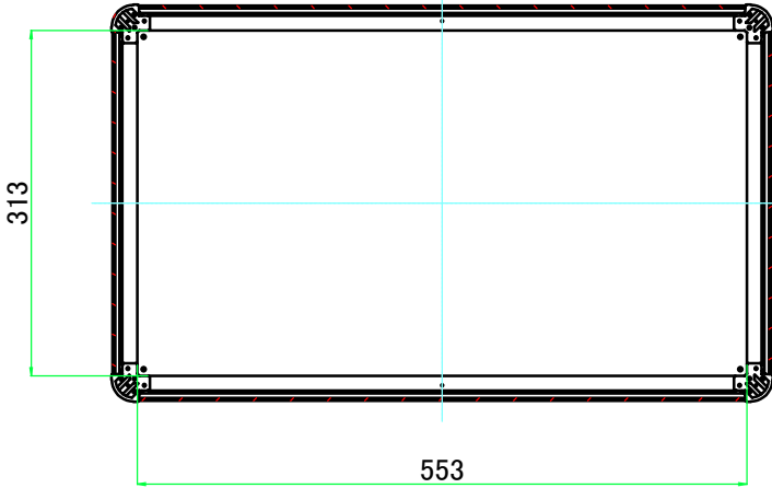
C-C ( 1 : 7.5 )
